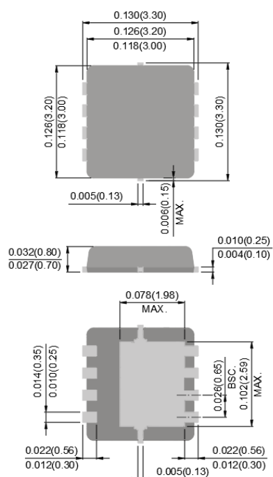
DFN3333-8L Dimension
