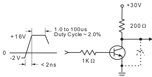
Fig. 1 Turn-On Time
