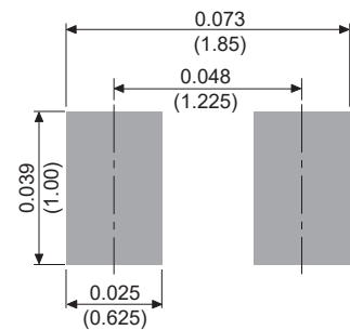
DFN1610-2L
