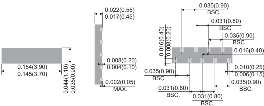
DFN3810-9L
