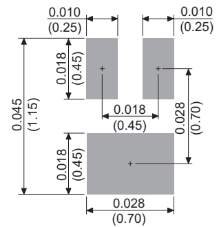
DFN1610-2L
